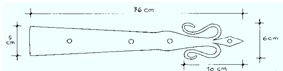
REFUERZO O FALSA BISAGRA DE LA PUERTA A LA HUERTA
