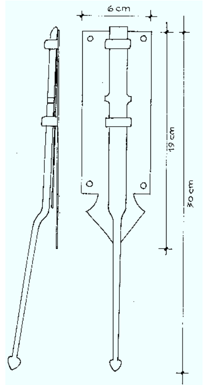
PASADOR SUPERIOR DE VENTANA Y BALCON
