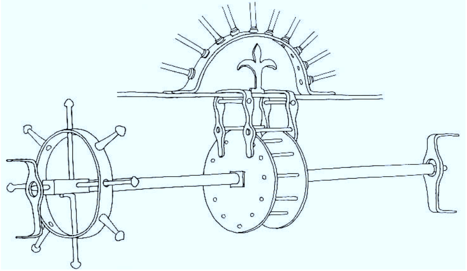
TORNO DEL ALGIBE
