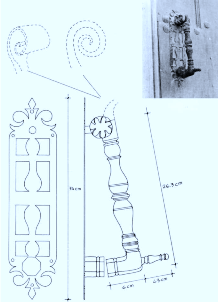
ESCUDO DE LA ALDABA
