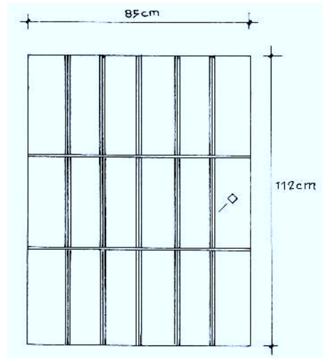
REJA DE VENTANA
