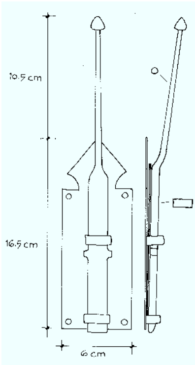
PASADOR INFERIOR DE VENTANA Y BALCON
