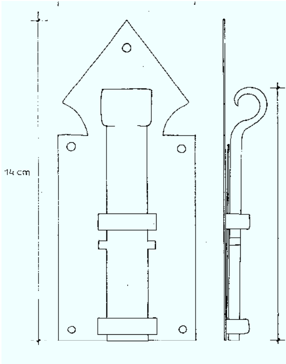
PASADOR INFERIOR Y SUPERIOR DE PUERTA DE BALCON
