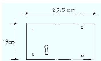
CERRADURA DE LA PUERTA DE LA SALA Fig. 176
