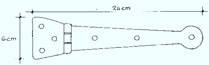
BISAGRA DEL BALCON
