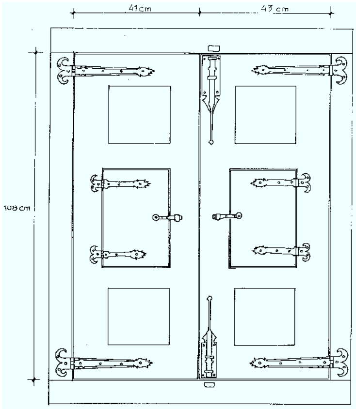
VENTANA CON SU HERRAJE VISTA INTERIOR
