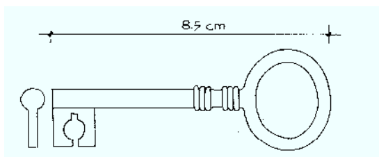
LLAVE Y BOCALLAVE DEL ARMARIO EMPOTRADO DE UNA HABITACION
