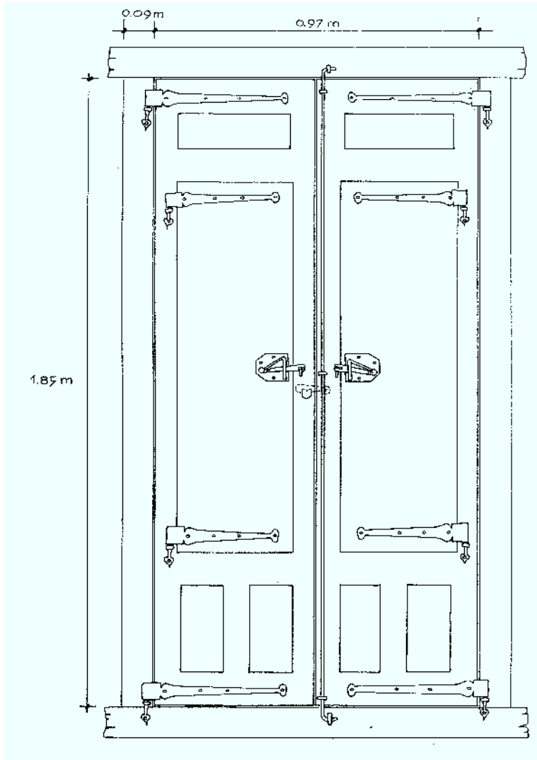
PUERTA DE BALCON CON SU HERRAJE VISTA INTERIOR
