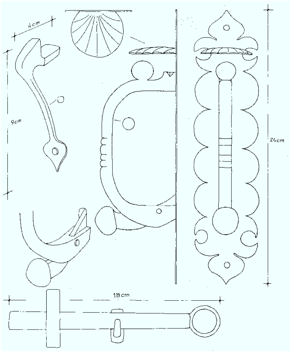
CRISQUETE DE LA PUERTA DE LA SALA
