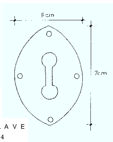
HERRAJES DE LA PUERTA DE SALA
