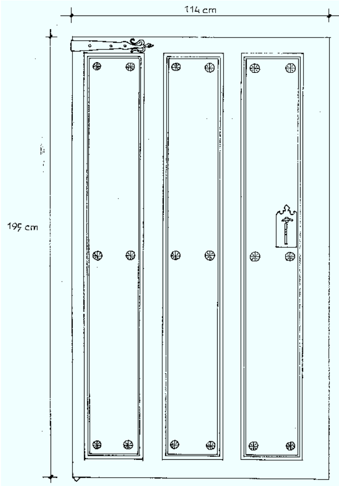
PUERTA A LA HUERTA Fig. 217
