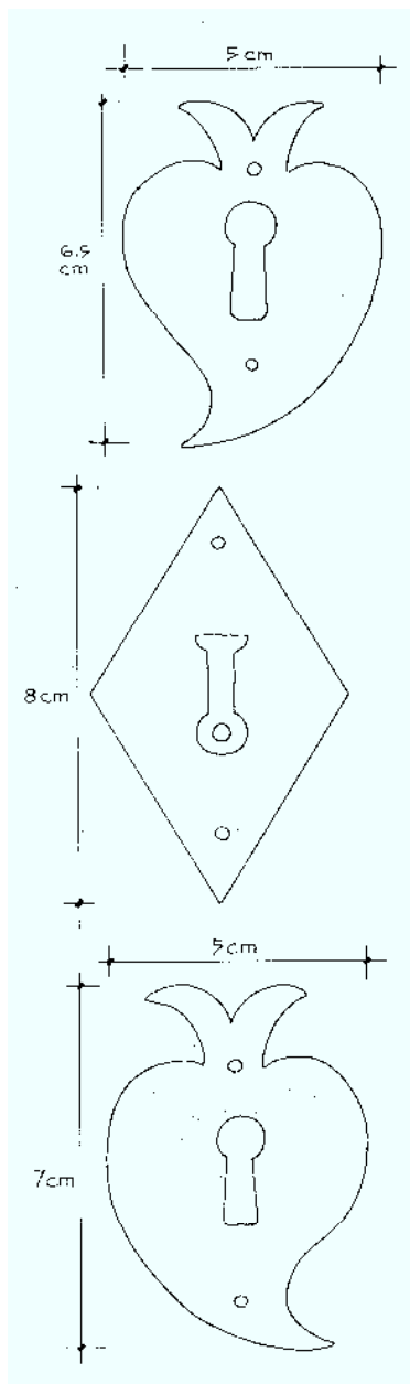
LLAVES Y BOCALLAVES DE LOS ARMARIOS EMPOTRADOS DE LA SALA
