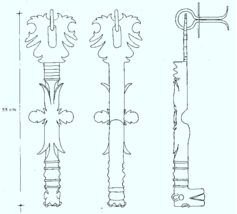
VISTA FRONTAL V. POSTERIOR V. LATERAL
