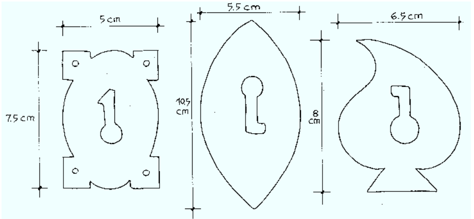
BOCALLAVE DE PUERTA DE HABITACION
