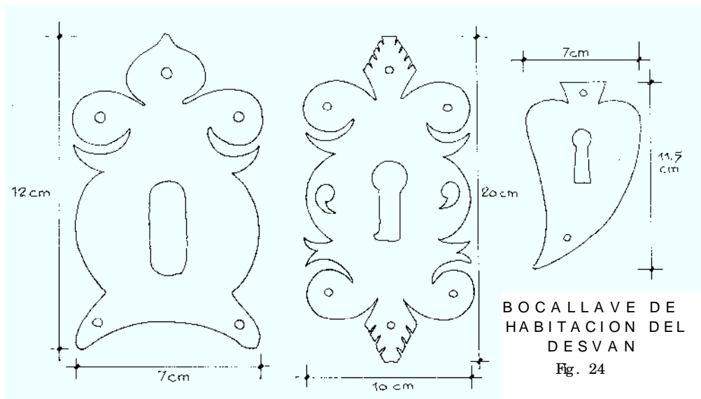
BOCALLAVE DE HABITACION DEL DESVÁN
