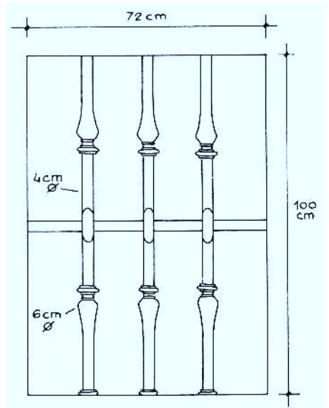
REJA DE VENTANA
