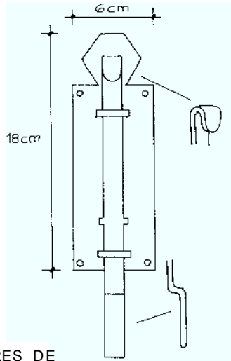
PASADORES DE LA PUERTA DE LA ESCALERA
