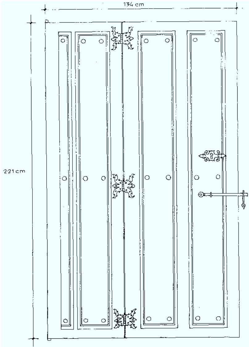
PUERTA DEL "PAYO"
