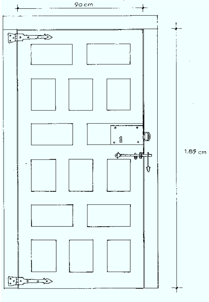
PUERTA DE HABITACION - SALA
