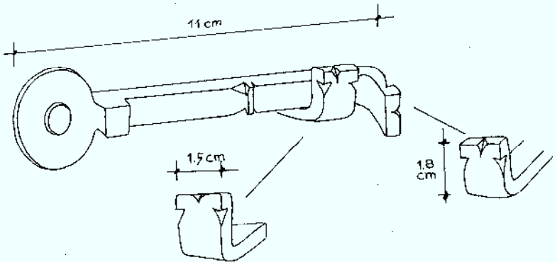
ALDABILLA DE CIERRE DEL VENTANILLO
