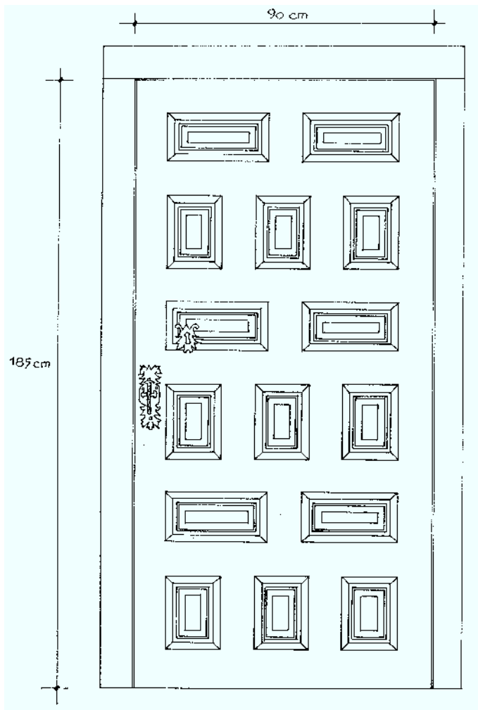
PUERTA DE HABITACION - SALA
