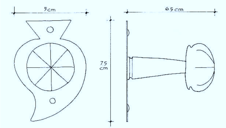
TIRADOR PUERTA PRINCIPAL
