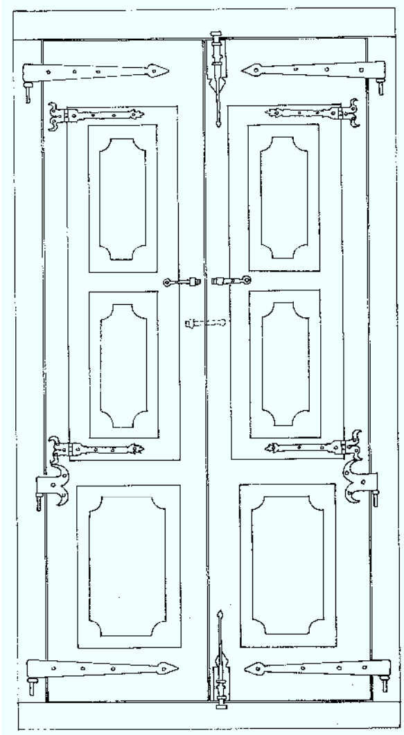
PUERTA DE BALCON CON SUS HERRAJES VISTA INTERIOR Fig. 179
