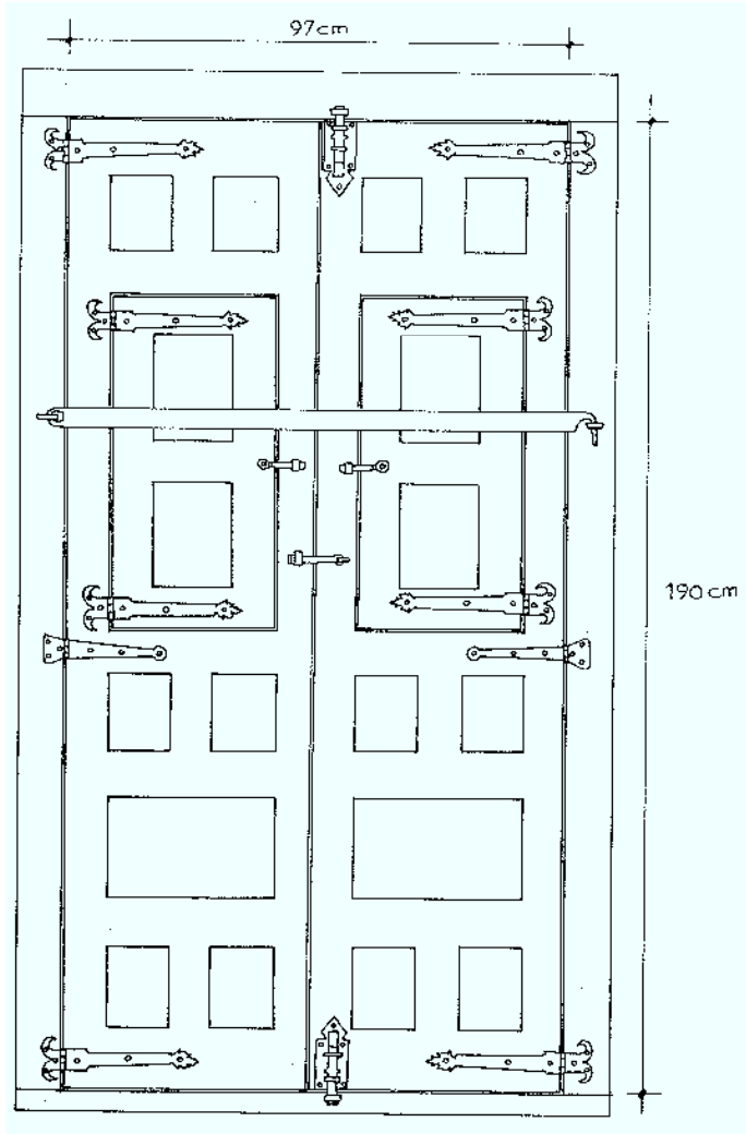
PUERTA DE BALCON CON SU HERRAJES VISTA INTERIOR
