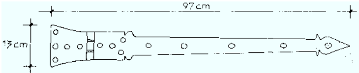
BISAGRA DE LA PUERTA DE CANCELA
