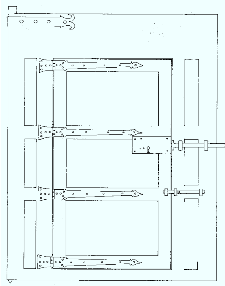
HERRAJE DE LA PUERTA PRINCIPAL (VISTA INTERIOR)
