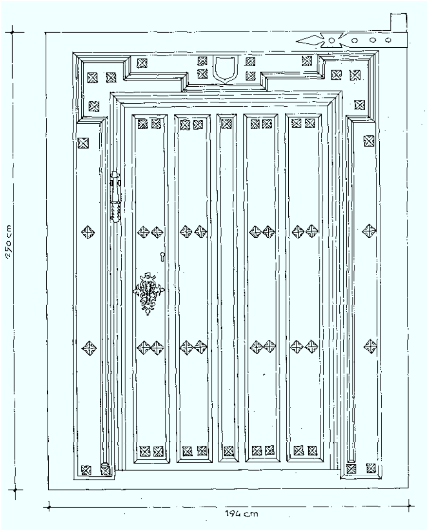
HERRAJE DE LA PUERTA PRINCIPAL (VISTA EXTERIOR)
