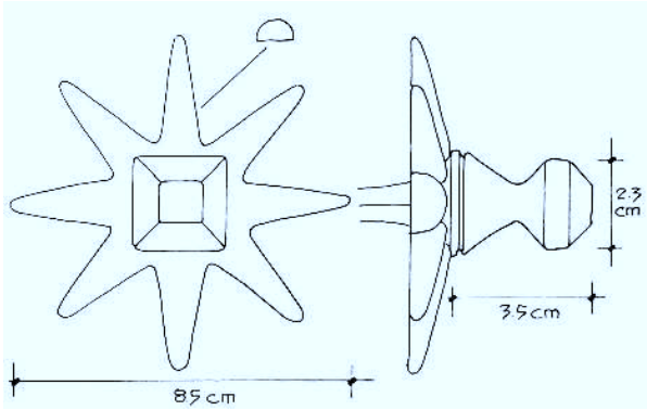
CLAVO DE LA PUERTA PRINCIPAL
