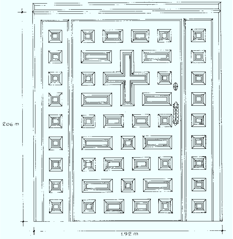
PUERTA DE SALA
