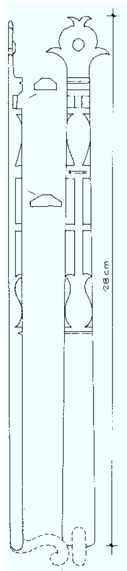
PIEZA DEL CRISQUETE DE LA PUERTA PRINCIPAL
