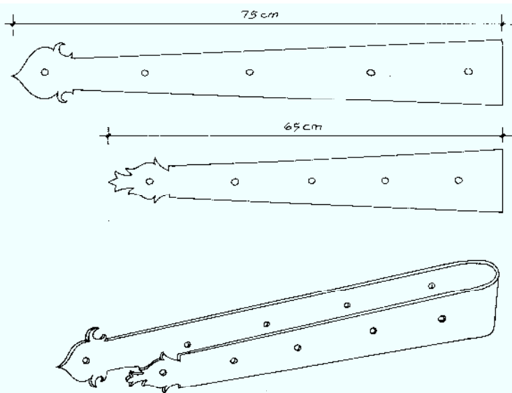
REFUERZO DE LA PUERTA PRINCIPAL
