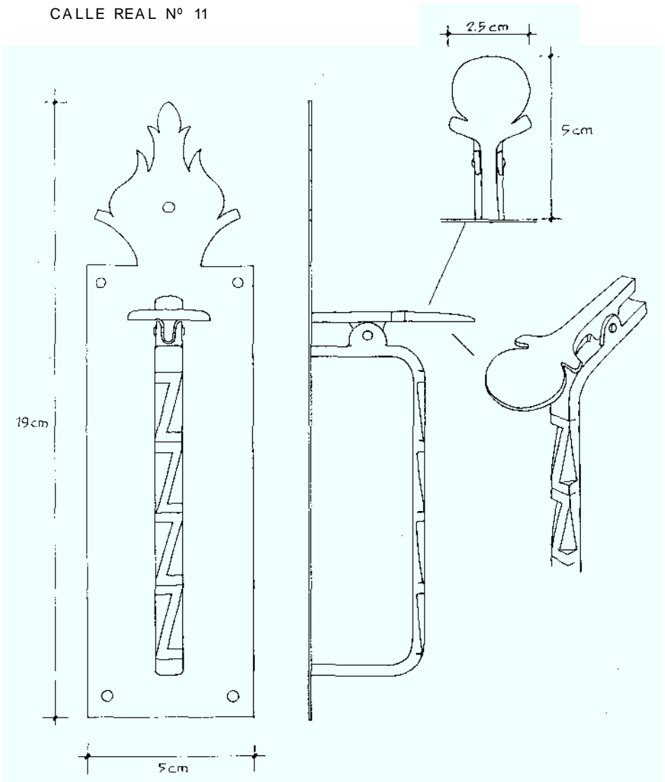
CRISQUETE DE PUERTA DE HABITACION
