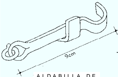
ALDABILLA DE CONTRAVENTANA Fig. 203 BIS
