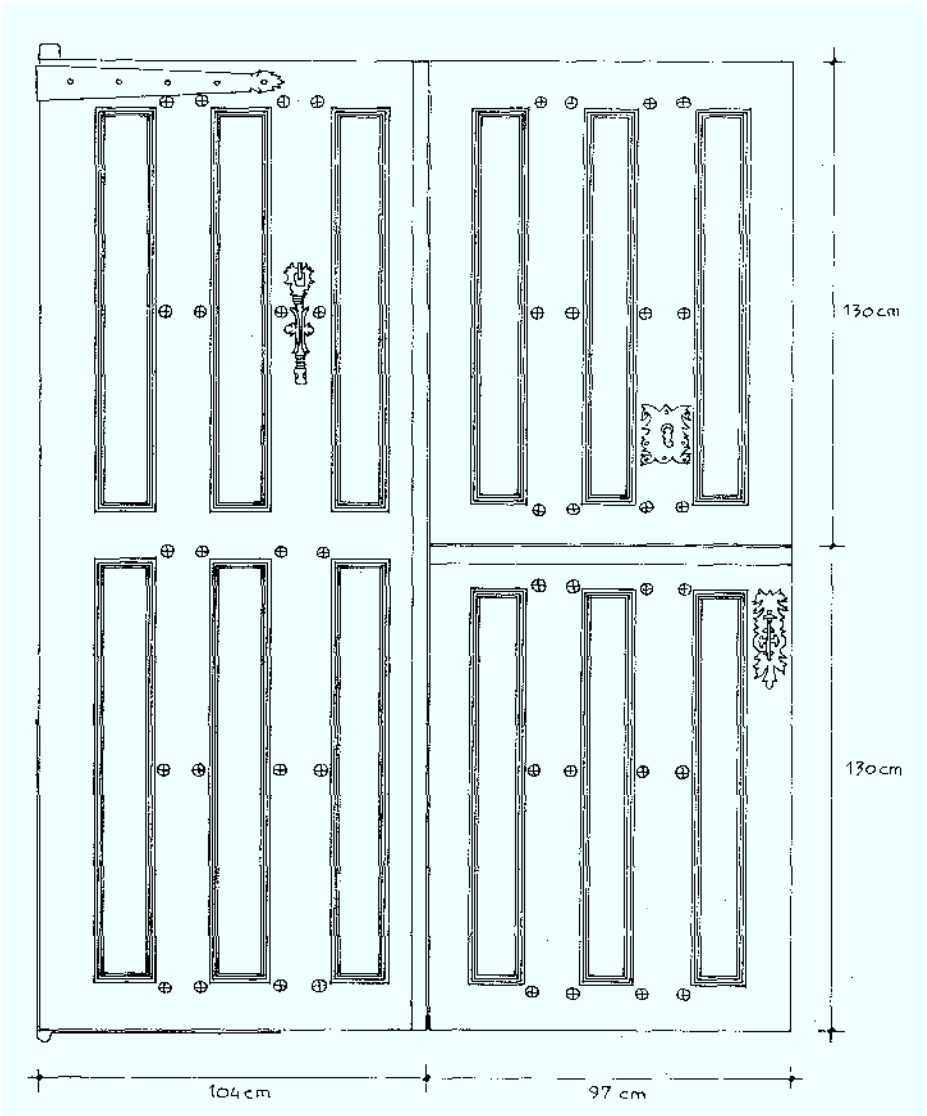
ALZADO DE LA PUERTA PRINCIPAL CON SUS HERRAJES VISTA EXTERIOR
