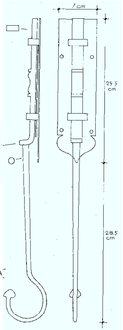
PASADOR SUPERIOR DE LA PUERTA DE LA E S C A L E R A
