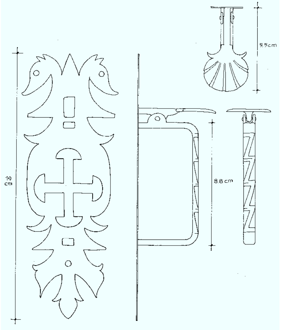
CRISQUETE DE PUERTA DE SALA
