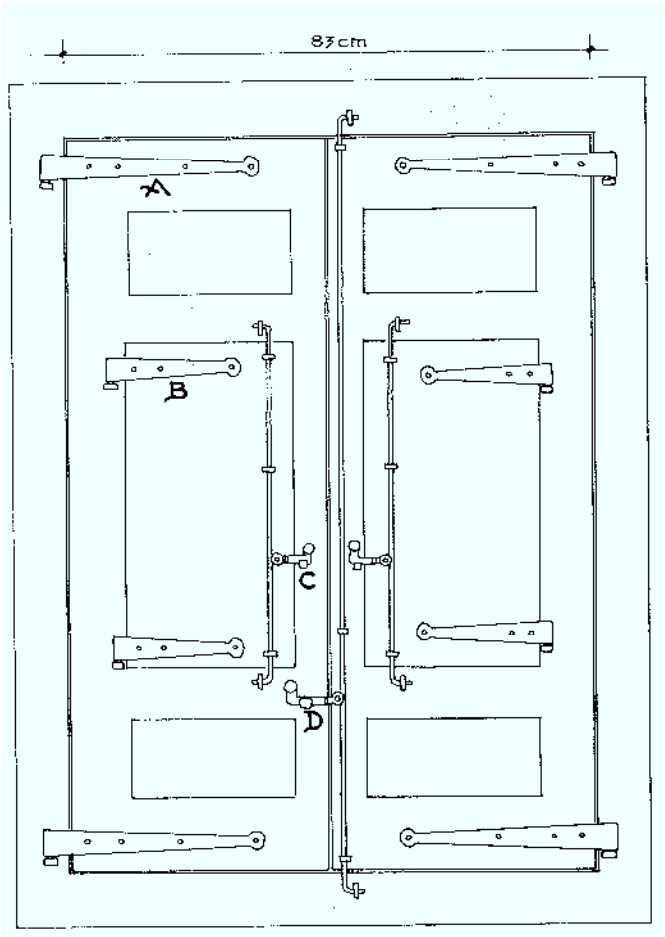
VENTANA CON SU HERRAJE VISTA INTERIOR Fig. 15
