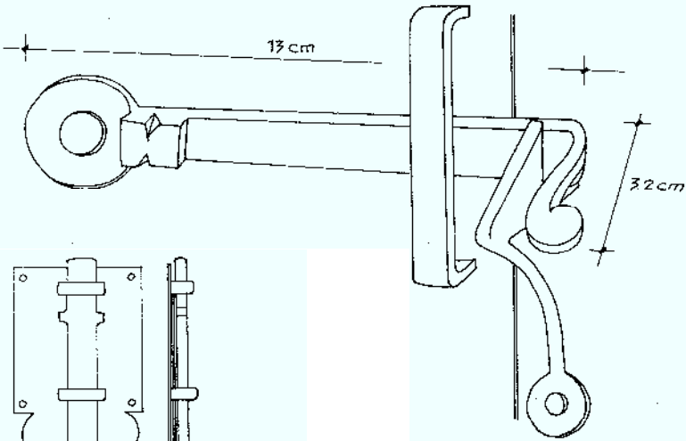
PICAPORTE DE PUERTA DE SALA
