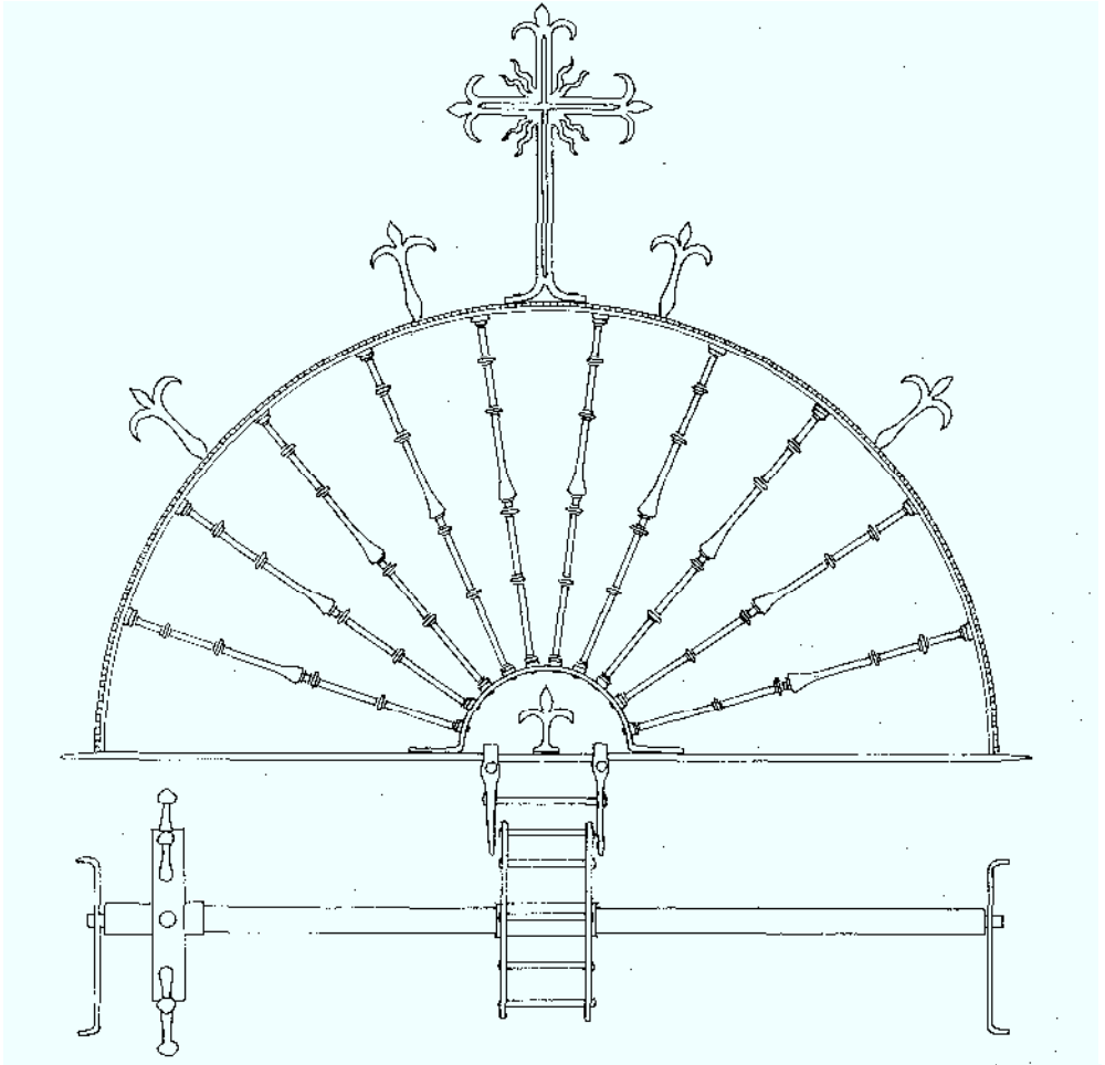
COPETE Y TORNO DEL ALGIBE
