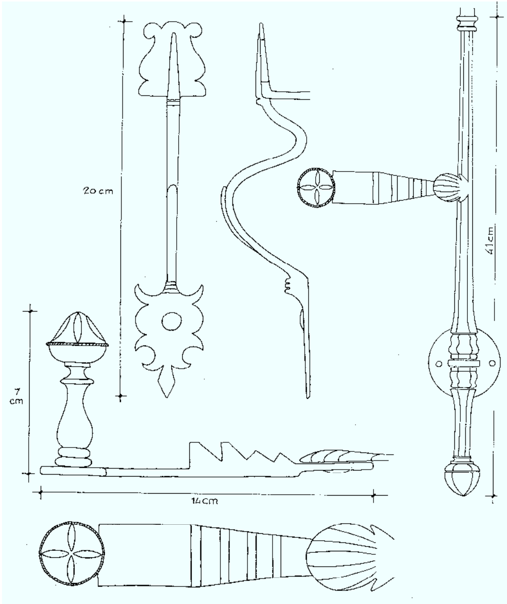
FALLEBA DE PUERTA DE BALCON
