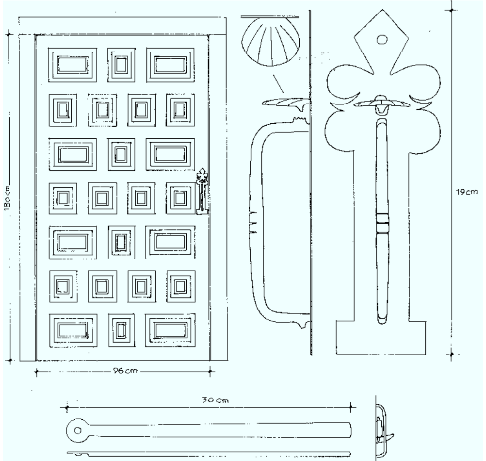
PUERTA DE HABITACION CON SU CRISQUETE
