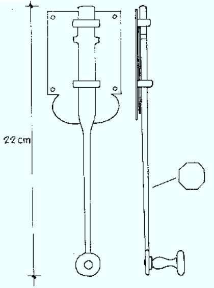
PICAPORTE DE PUERTA DE SALA
