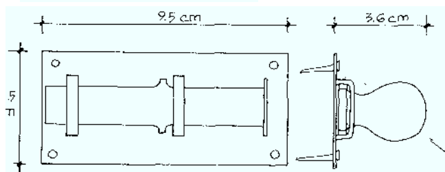
CERRADURA DE LA PUERTA DE LA SALA Fig. 176
