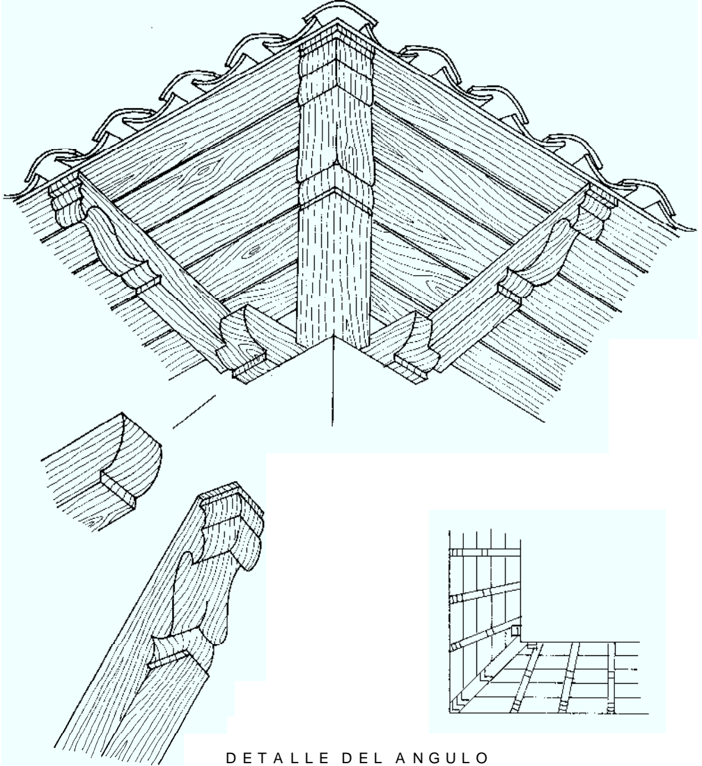
DETALLE DEL ANGULO DEL ALERO
