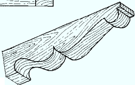
CAN DE ALERO DE FACHADA LATERAL
