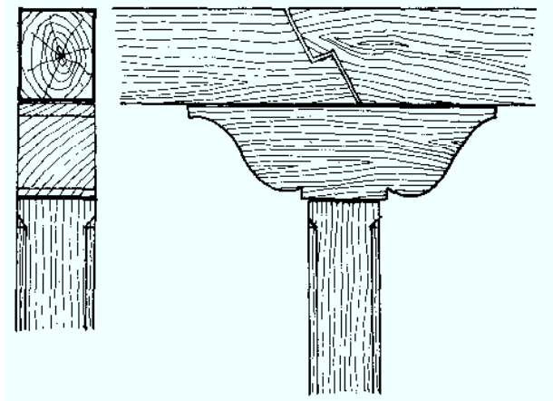
ZAPATA DEL TEJADILLO DEL BALCON
