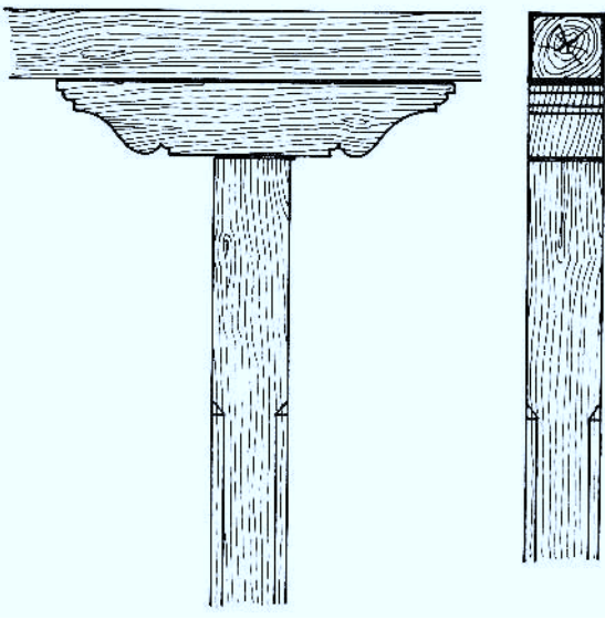
POSTE Y ZAPATA DEL TEJADILLO DEL BALCON
