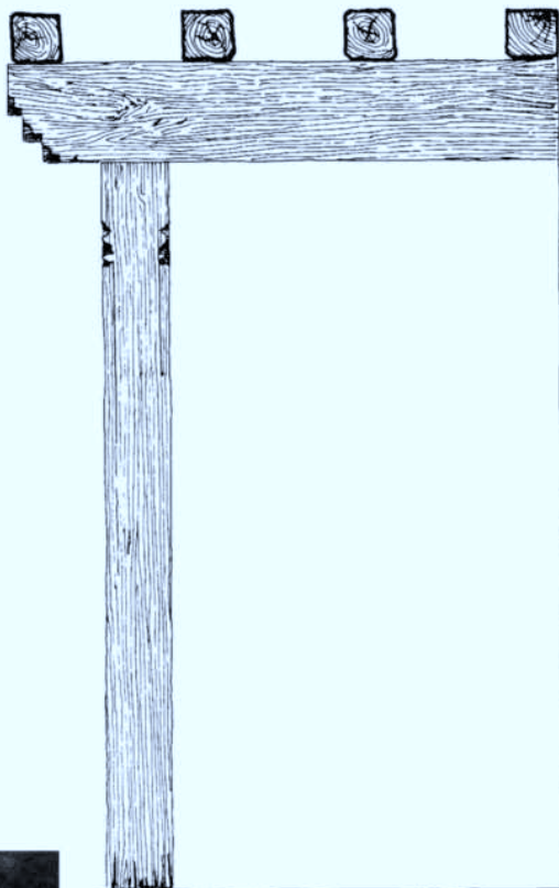
DETALLES DE LA TESTA DE LA VIGA A
