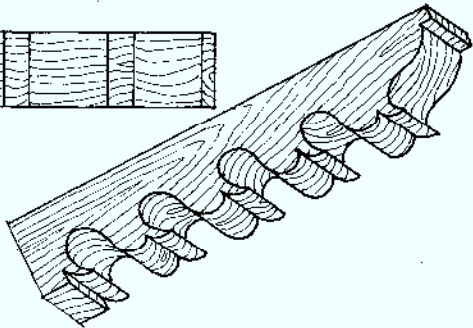
CAN DE ALERO DE FACHADA PRINCIPAL
