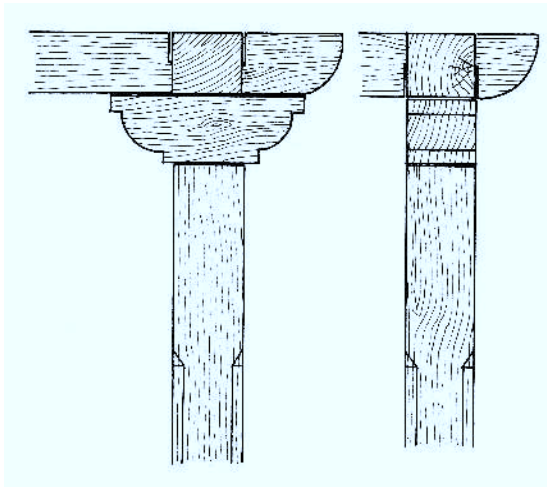
POSTE Y ZAPATA DE ANGULO DEL TEJADILLO DEL BALCON.
