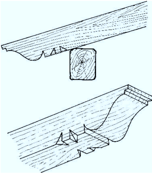
TALLA EN EL EXTREMO DE LOS CABIOS DEL PORTICO
