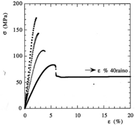
11 irudia. Konpositeen tentsio-deformazio kurbak: (○) PES, (+) CPES 10, (□) CPES 20, (■) CPES 30
