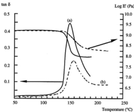
13 irudia. Kristaltasun desberdineko PEEK hutsaren espektro mekanikoak (maiztasuna 1 Hz) (a) X_c = 14\% (EKD) (b) X_c = 30\% (EKD)
