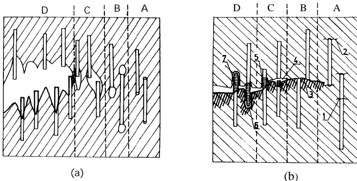
27 irudia. Pitzaduraren hedapena bi deformazio-mekanismo desberdinen bitartez: (a) ebakidura eta (b) mikropitzadura.
