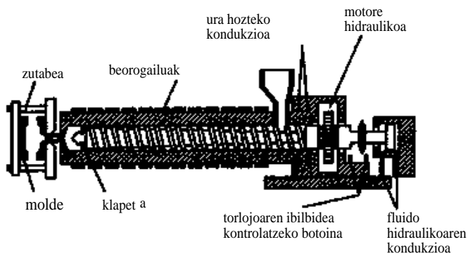
4 irudia. Zizta-moldeaketa makina
