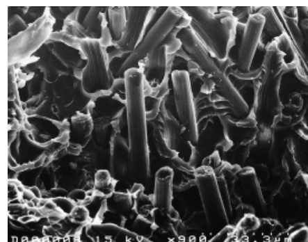
(d) PES/CF
