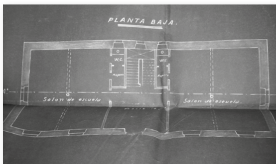
Eskola zaharren lehen solairuaren plano / Plano de la planta baja de las escuelas viejas de Urduliz. 1897. BFAH/AHFB AR 00173/001
