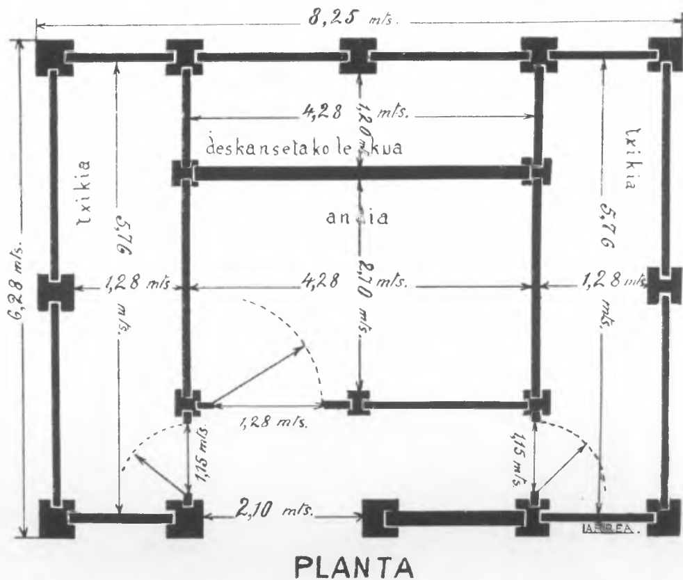
Fig. 2.—Planta del garaixe del caserío Zenita-aldekua.
