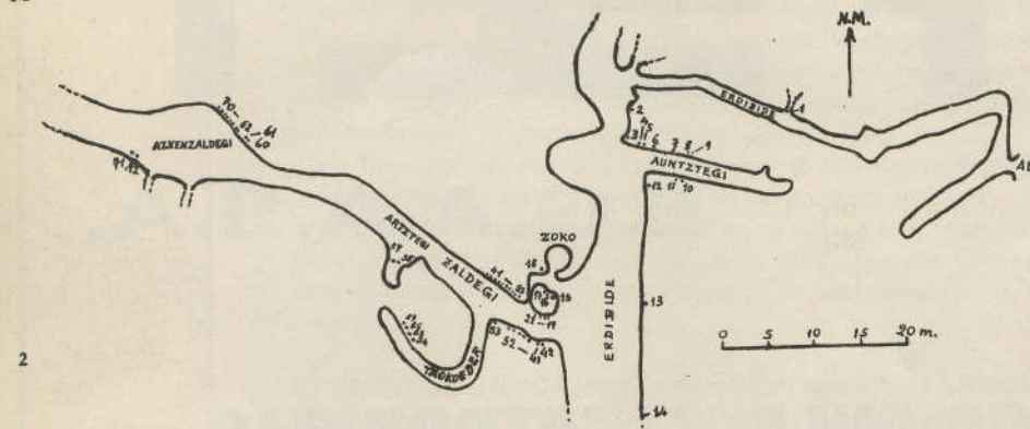
Planta topográfica de la Cueva de Ekain.
